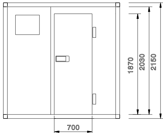
Zij aanzicht
