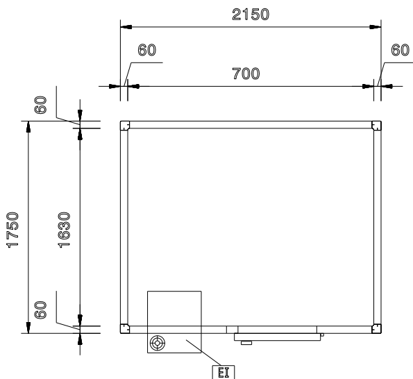
Zij aanzicht
